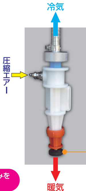
暖気の風量調整弁。 これで冷風の風量と温度を変える
